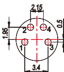
4针、母头
