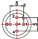
5针、母头
