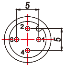
4针、母头
