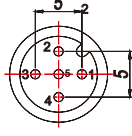
5针、母头
