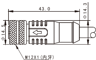
M12 母头,直头,屏蔽
