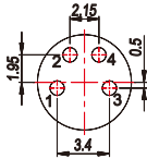
4针、母头
