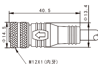
M12 母头,直头
