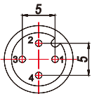
4针、母头
