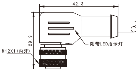
M12 母头,弯头,带LED灯,NPN
